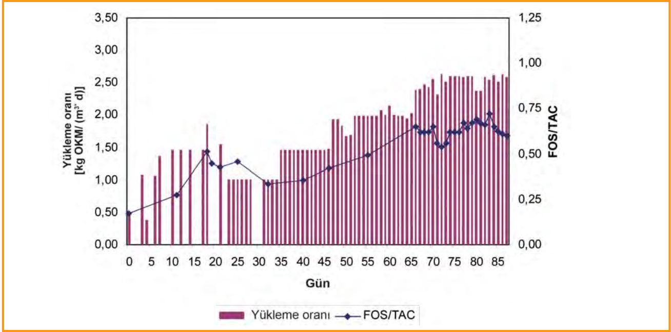
Şekil 5.4: Başlatma aşaması fermentör 1
