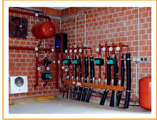
Şekil 6.7: Isı dağıtıcısı [MT-Energie-GmbH]
